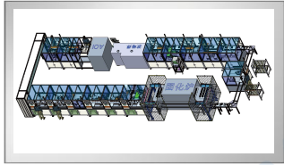
汽车水加热器模块智能产线 Auto water heater module intelligent production line
